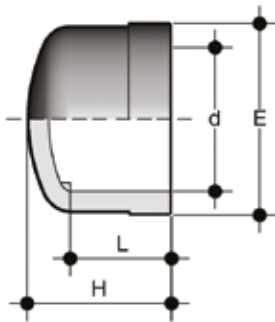
CIV Endkappe mit Klebemuffe
