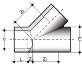
YIV 45° T-Stück mit Klebemuffe
