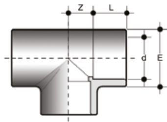
TIV 90° T-Stück mit Klebemuffe
